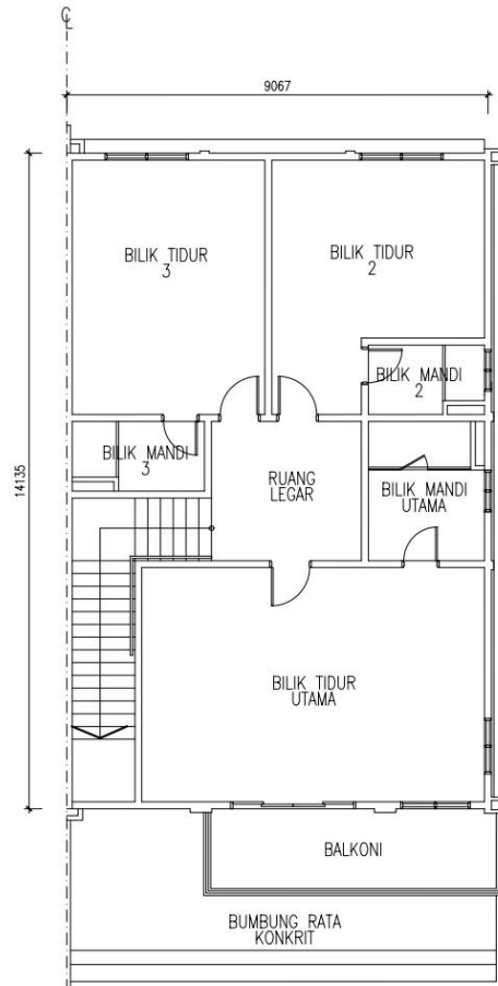
ARAS ATAS
