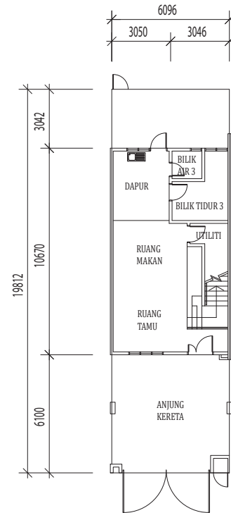
JENIS RT3 PELAN TINGKAT BAWAH
