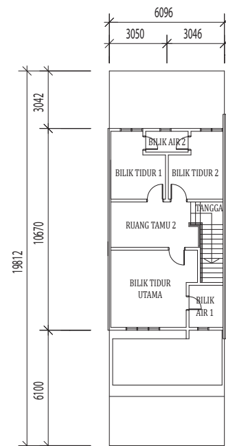
JENIS RT3 PELAN TINGKAT SATU
