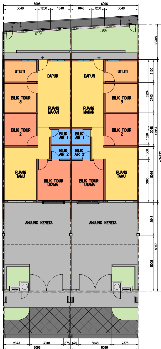
PELAN LANTAI RUMAH TERES (4 BILIK)
