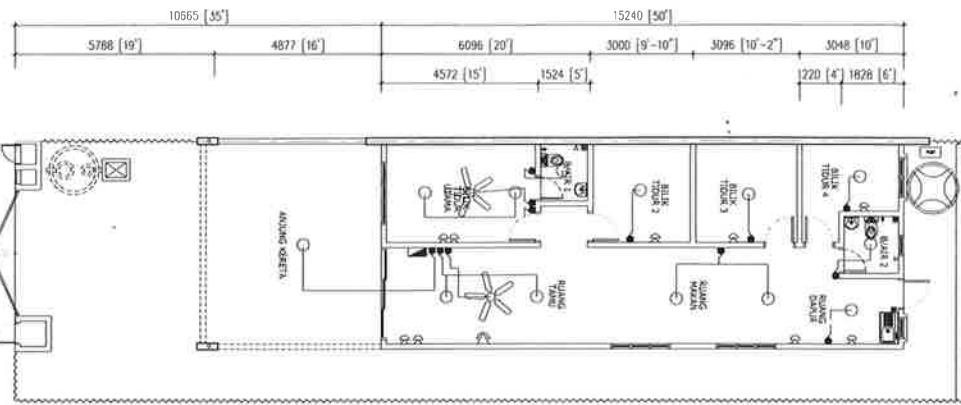
PELAN LANTAI
