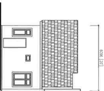
PANDANGAN BELAKANG
