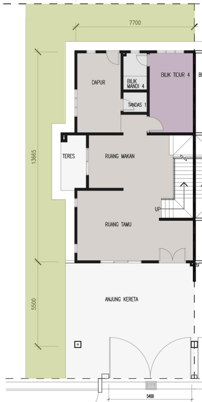
PELAN LANTAI TINGKAT 1
