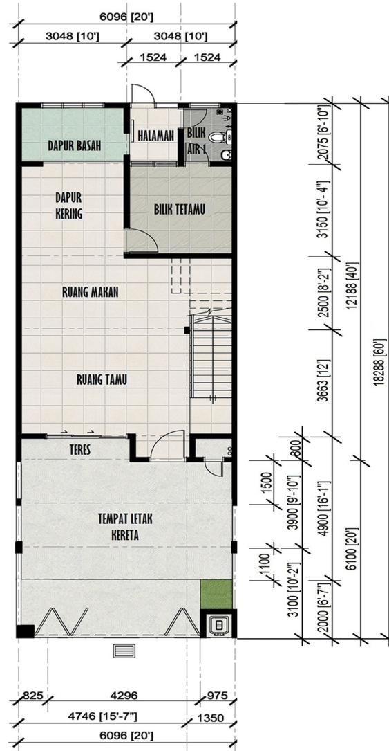
PELAN LANTAI TINGKAT BAWAH
