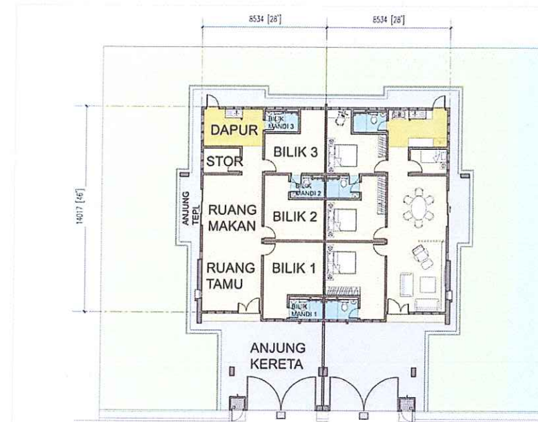
PELAN LANTAI
