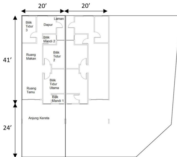
Pelan Lantai
