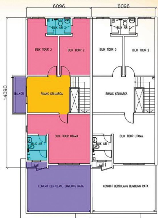
Pelan Lantai Aras Satu
