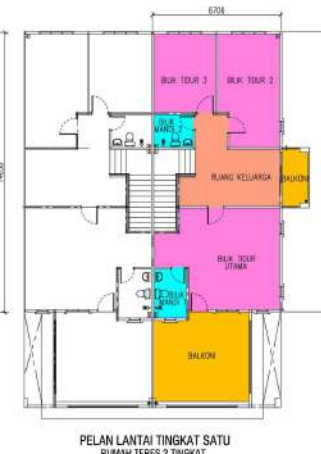
PELAN LANTAI TINGKAT SATU RUMAH TERES 2 TINGKAT
