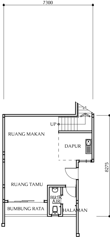
PELAN TINGKAT 1
