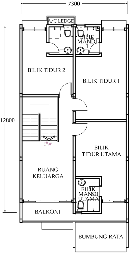
PELAN TINGKAT 2
