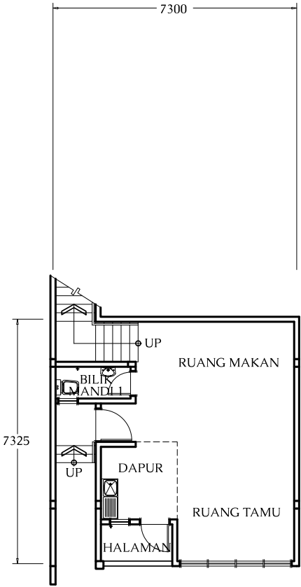
PELAN TINGKAT 1
