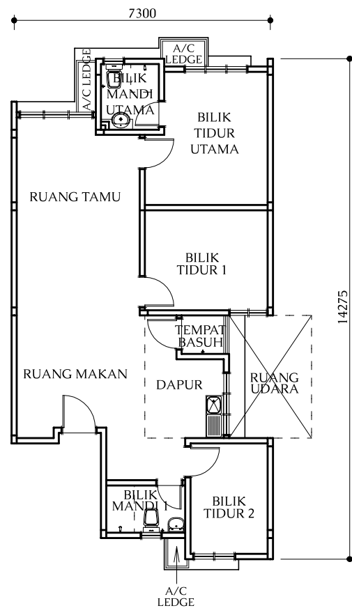
PELAN TINGKAT 1 & 2
