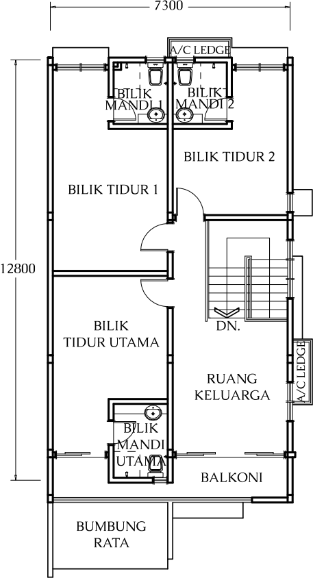
PELAN TINGKAT 2
