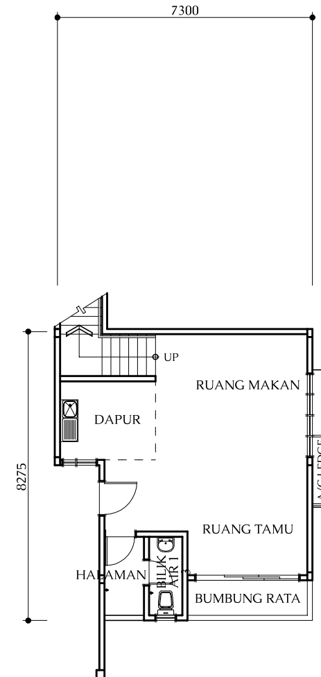
PELAN TINGKAT 1
