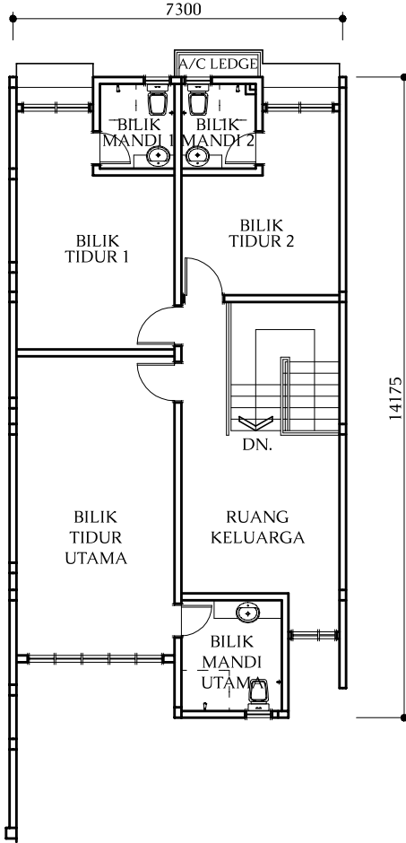
PELAN TINGKAT 2
