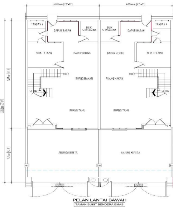
PELAN LANTAI – RUMAH TERES 2 TINGKAT TINGKAT BAWAH
