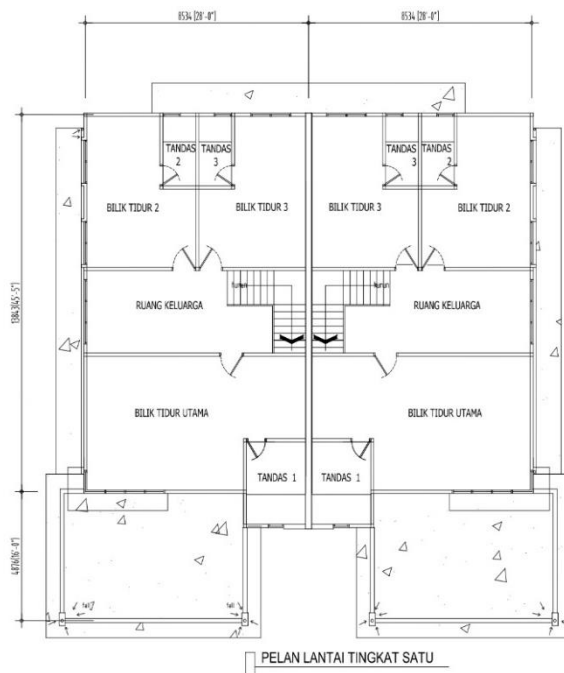
PELAN LANTAI – RUMAH BERKEMBAR 2 TINGKAT TINGKAT ATAS
