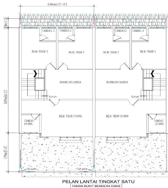
PELAN LANTAI – RUMAH TERES 2 TINGKAT TINGKAT BAWAH
