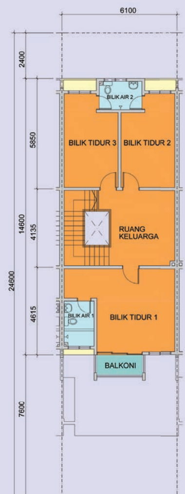
Pelan Tingkat Dua
