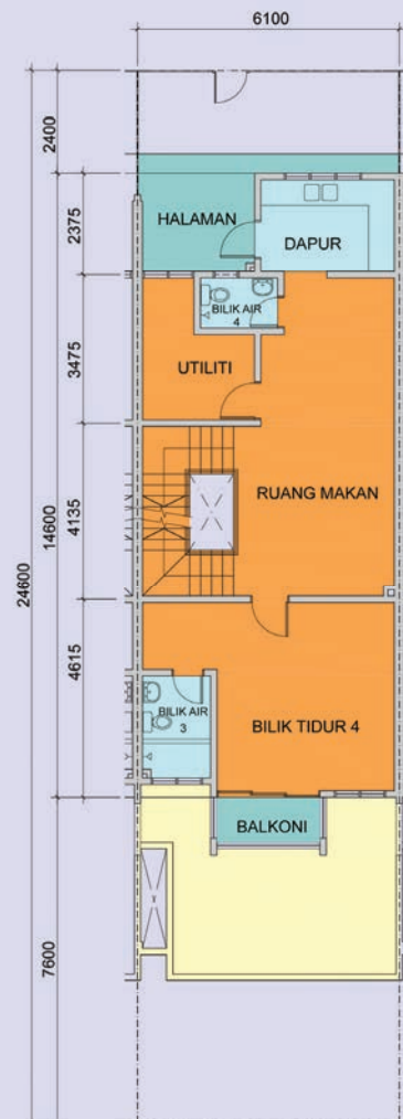
Pelan Tingkat Satu
