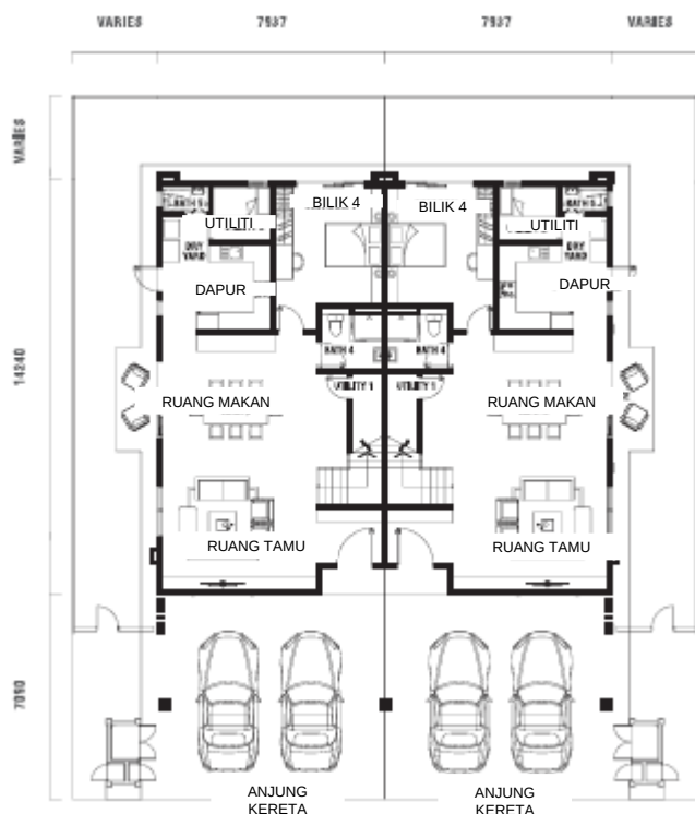
Tingkat Bawah
