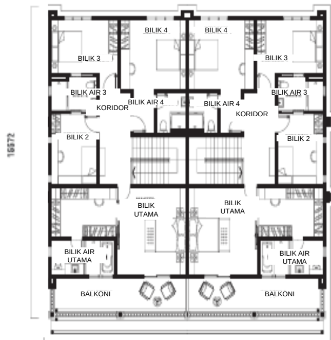
Tingkat Atas
