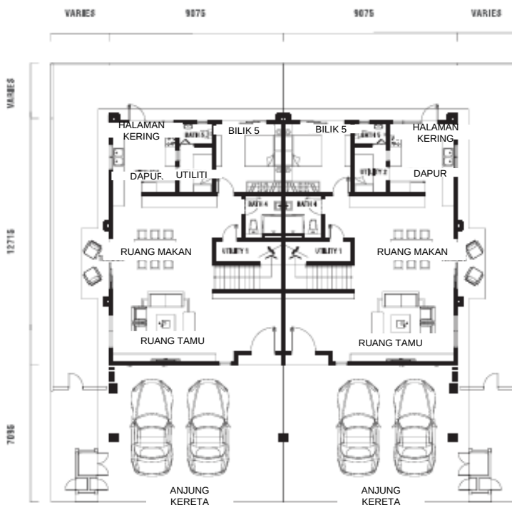
Tingkat Bawah
