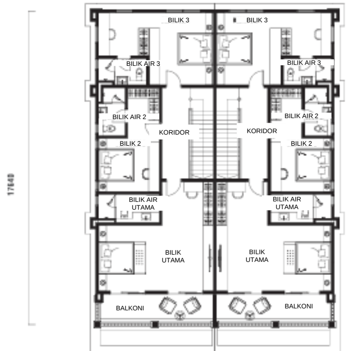
Tingkat Atas
