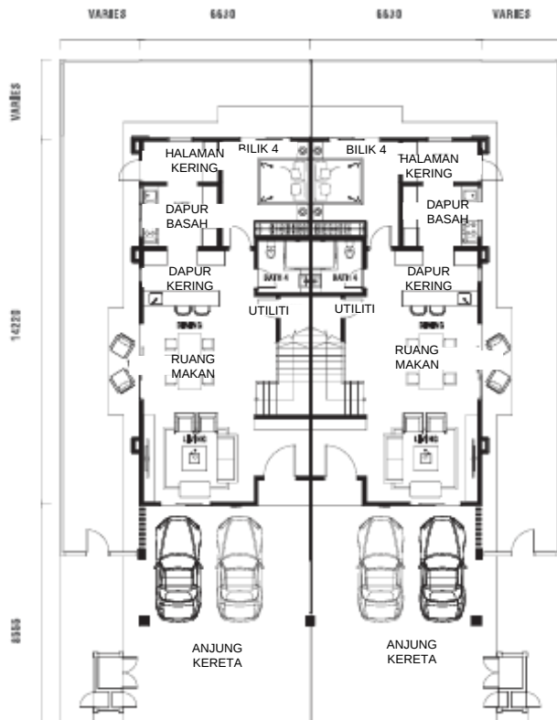
Tingkat Bawah
