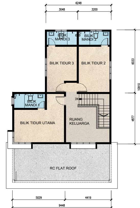
Tingkat Atas
