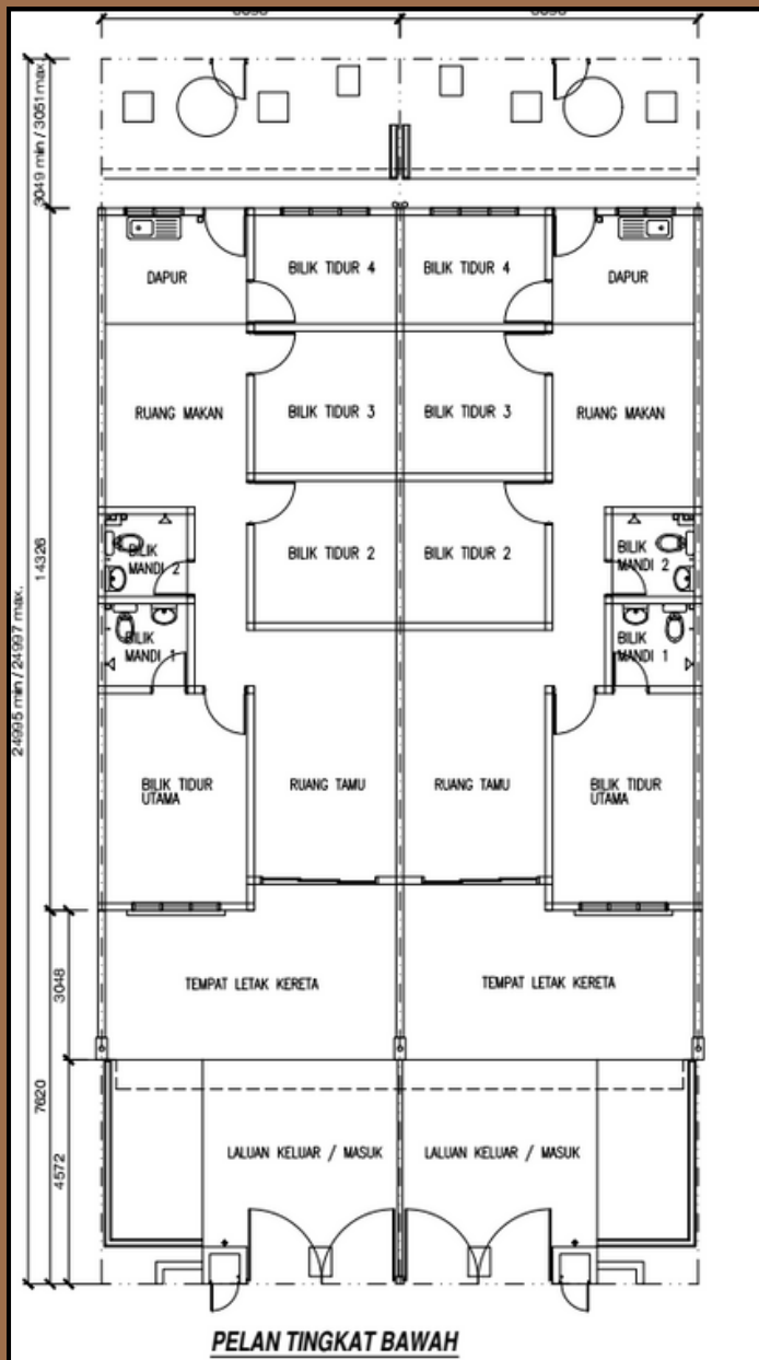
PELAN LANTAI RUMAH TERES 1 TINGKAT (20' X 47')
