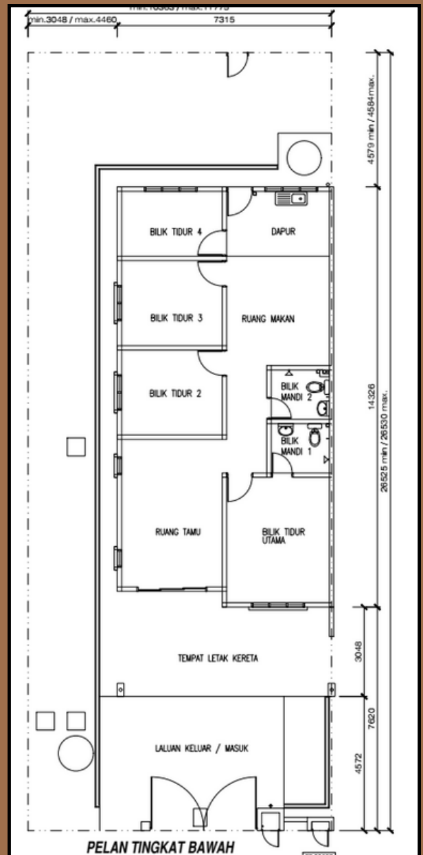
PELAN LANTAI RUMAH BERKEMBAR 1 TINGKAT (24' X 47')
