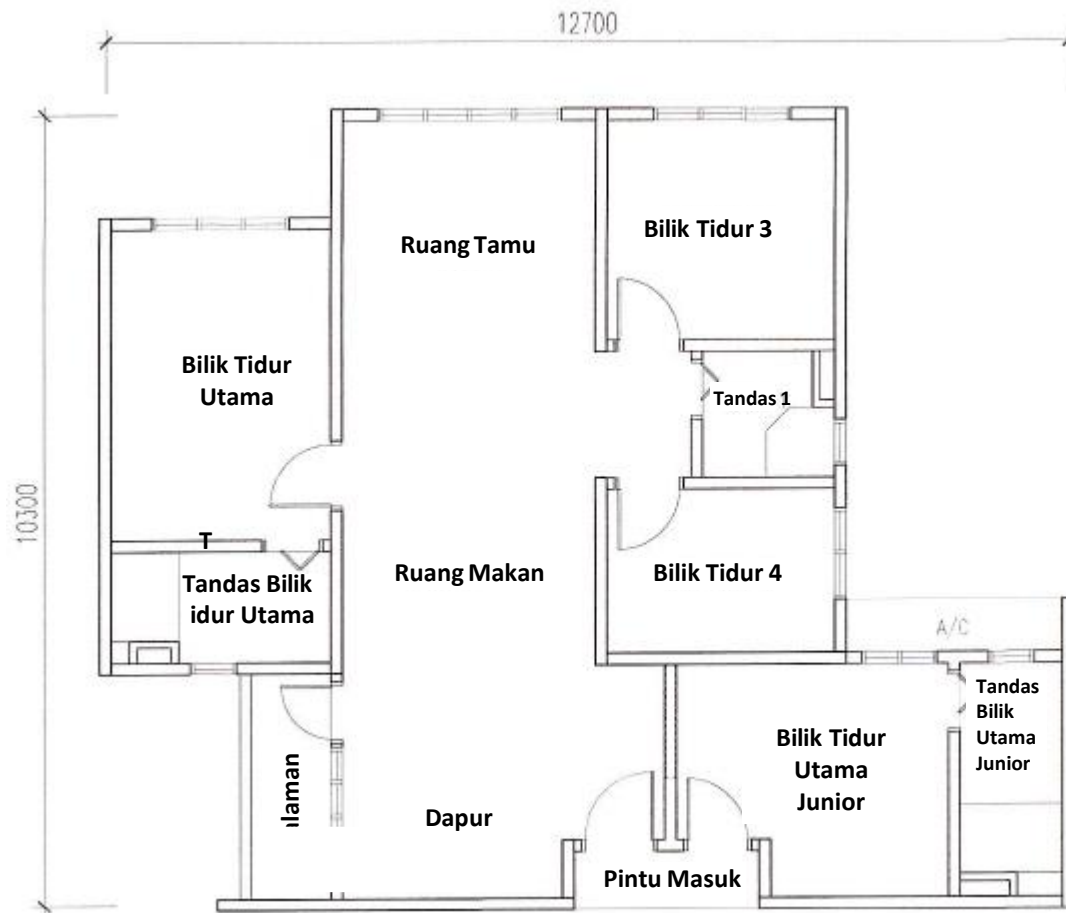
JENIS C DWI KUNCI (4 BILIK) – 100 m 2
