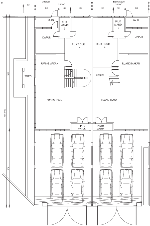
PELAN ARAS BAWAH
