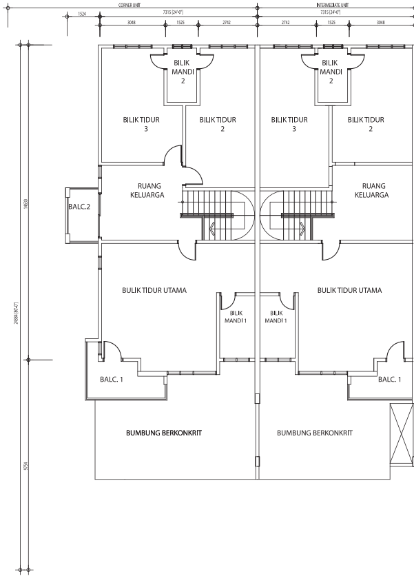
PELAN ARAS SATU
