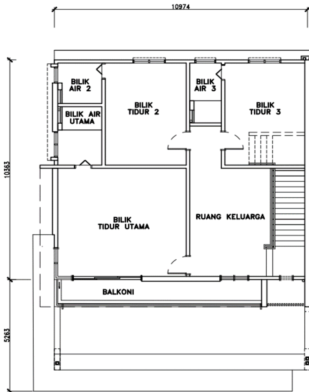
PELAN LANTAI TINGKAT ATAS
