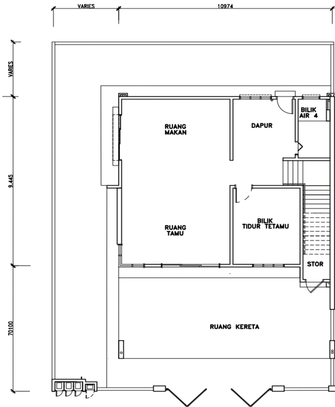
PELAN LANTAI TINGKAT BAWAH
