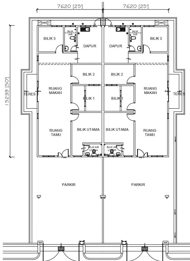
Pelan Lantai
