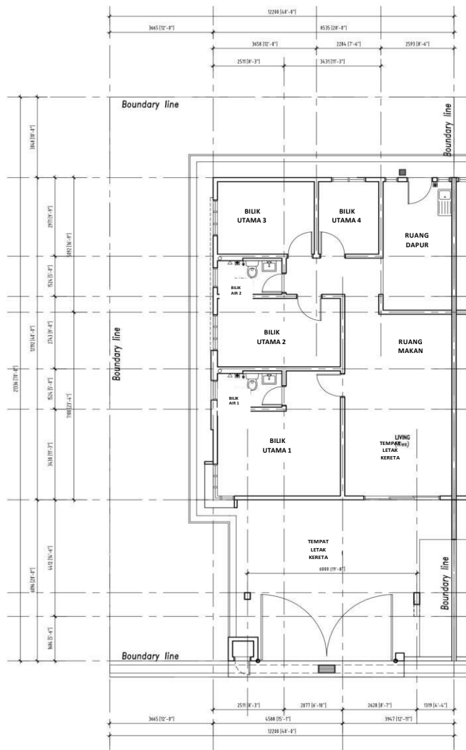
PELAN LANTAI BAWAH (KLUSTER JENIS C)
