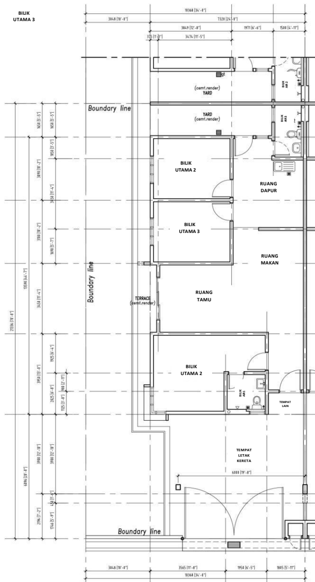
PELAN LANTAI BAWAH (KLUSTER JENIS A)
