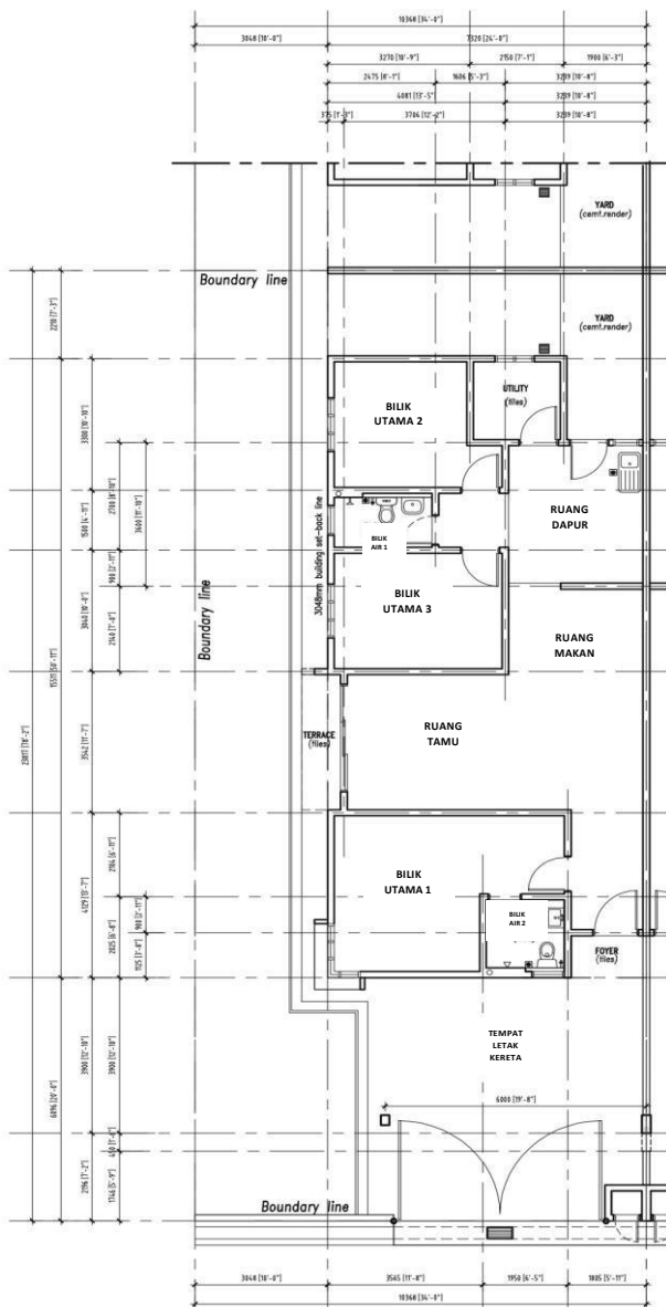
PELAN LANTAI BAWAH (KLUSTER JENIS B)
