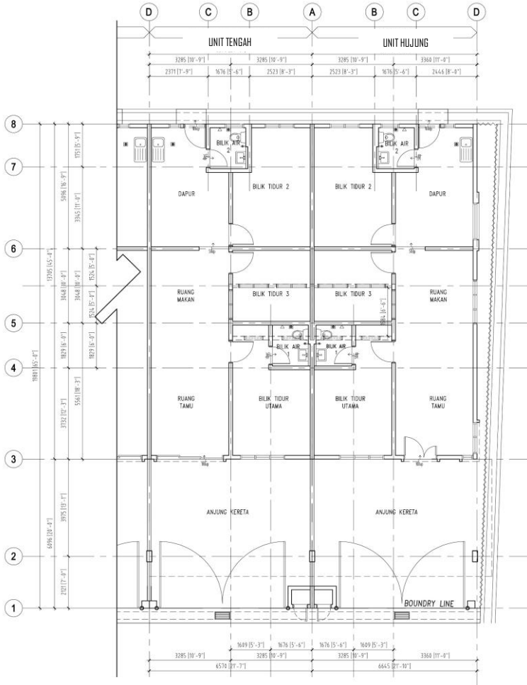
PELAN LANTAI
