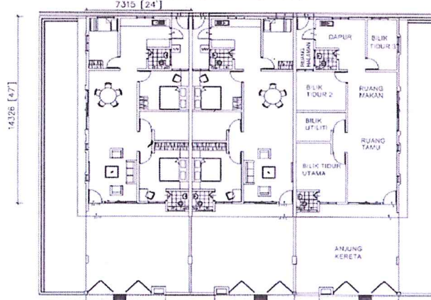
PELAN LANTAI RUMAH TERES 1 TINGKAT 24' X 47' (JENIS C)
