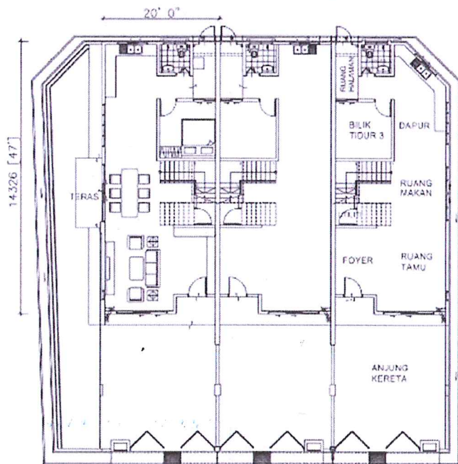
TINGKAT BAWAH PELAN LANTAI RUMAH TERES 2 TINGKAT 20' X 47' (Tingkat Bawah) / 20' x 50' (Tingkat Atas)
