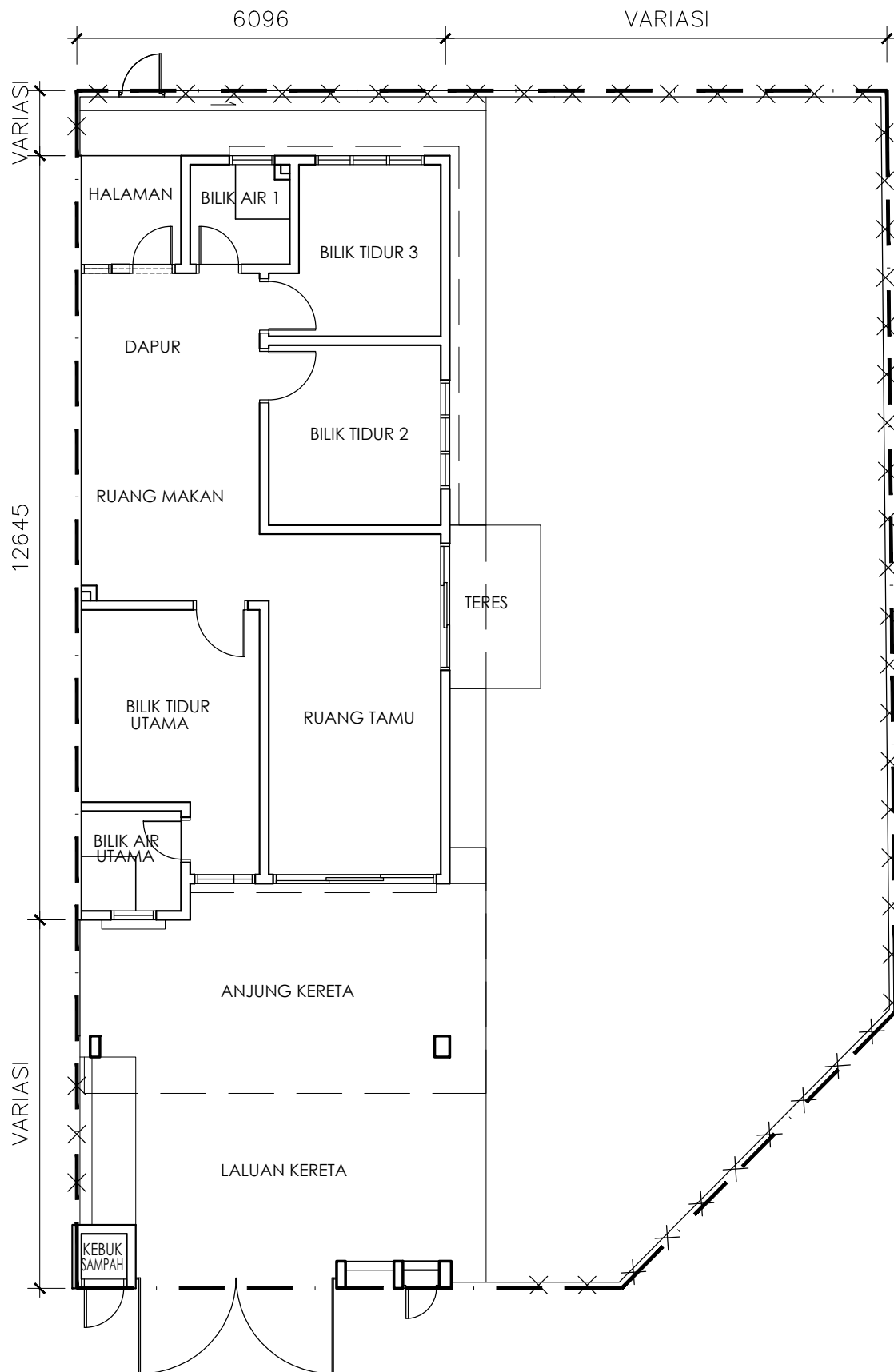
PELAN TINGKAT BAWAH
