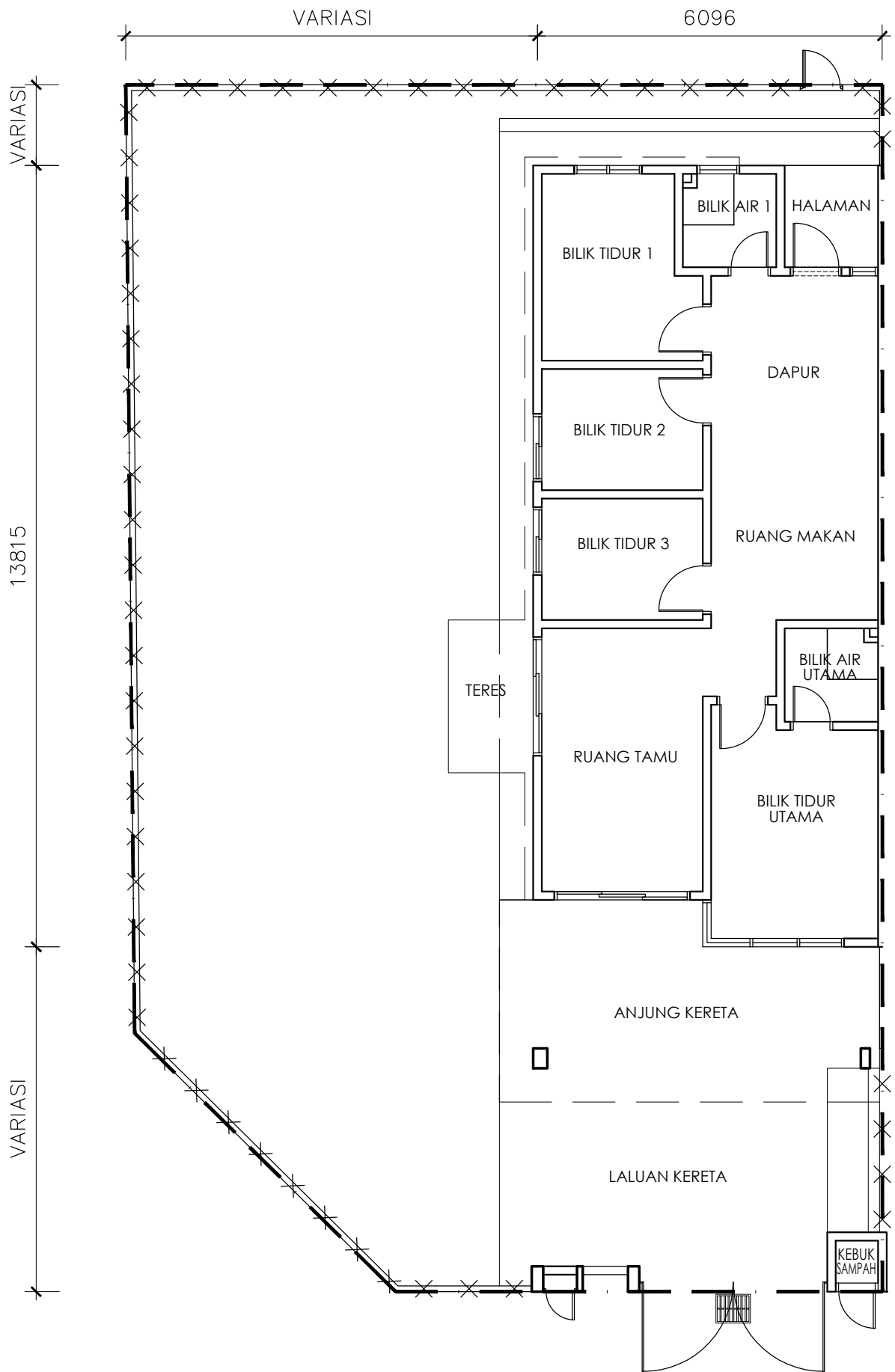
PELAN TINGKAT BAWAH
