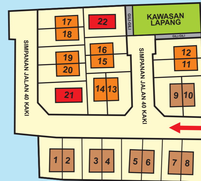
RUMAH BERKEMBAR SETINGKAT JENIS A (10 UNIT) LUAS TANAH (MIN) : 35' X 76' LUAS BINAAN : 27' X 42'
