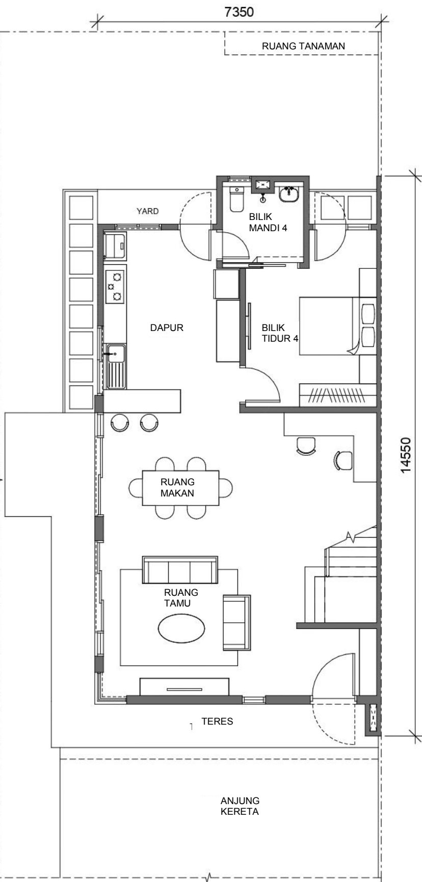
PELAN TINGKAT BAWAH
