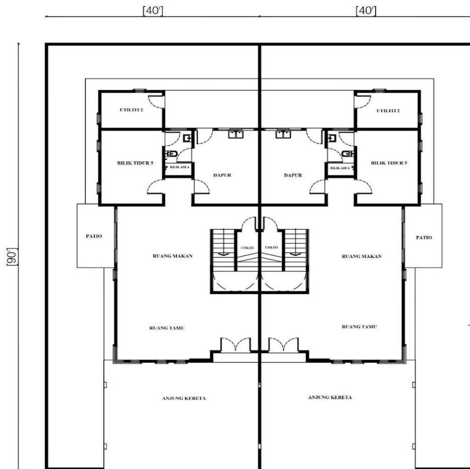
RUMAH BERKEMBAR 2 TINGKAT (40' X 90') - TINGKAT BAWAH
