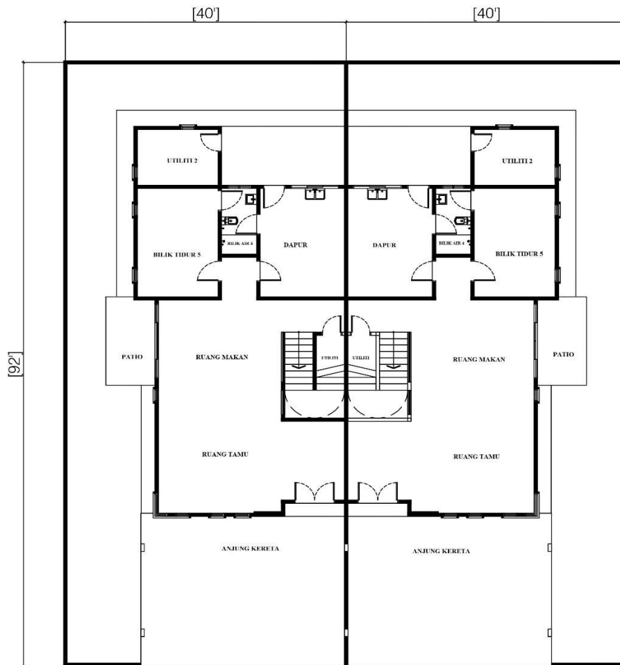
RUMAH BERKEMBAR 2 TINGKAT (40' X 92') - TINGKAT BAWAH
