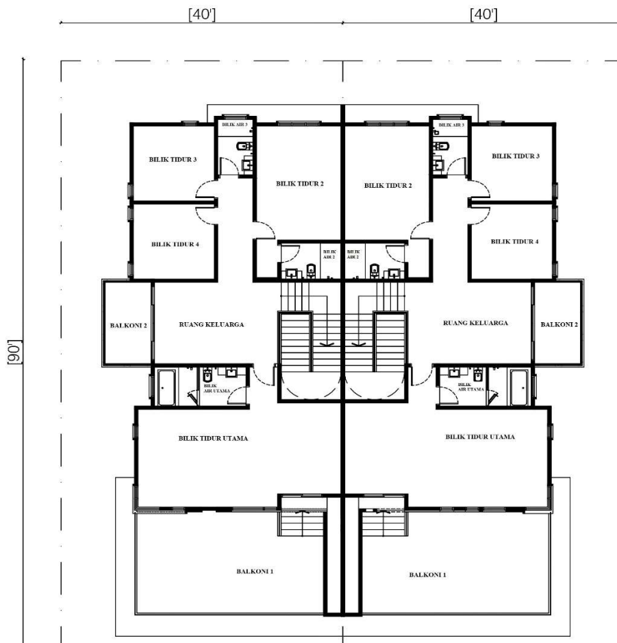
RUMAH BERKEMBAR 2 TINGKAT (40' X 90') - TINGKAT ATAS
