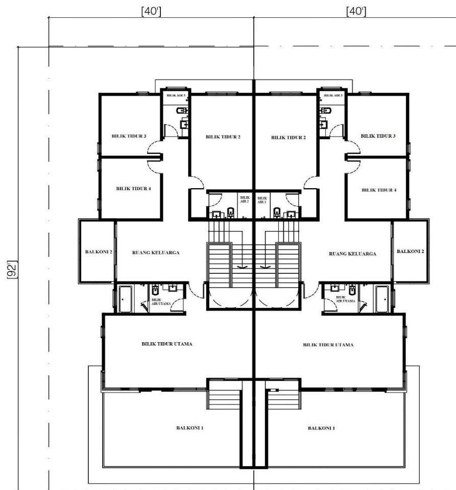
RUMAH BERKEMBAR 2 TINGKAT (40' X 92') - TINGKAT ATAS
