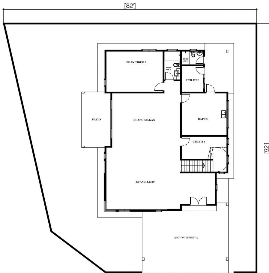
RUMAH BANGLO 2 TINGKAT - TINGKAT BAWAH
