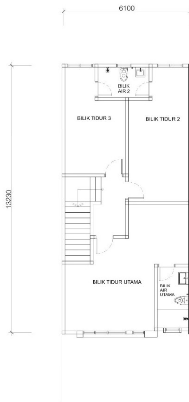
PELAN LANTAI TINGKAT ATAS
