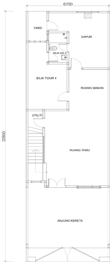
PELAN LANTAI TINGKAT BAWAH
