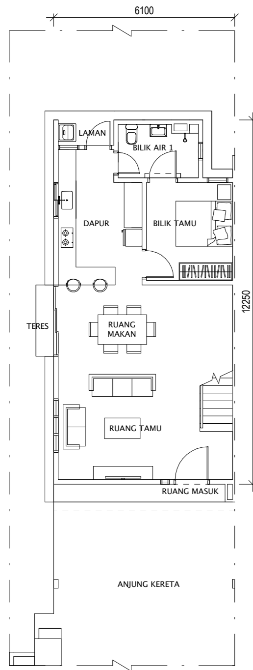
TINGKAT BAWAH
