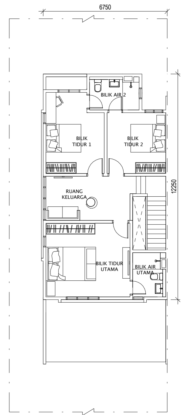
TINGKAT SATU
