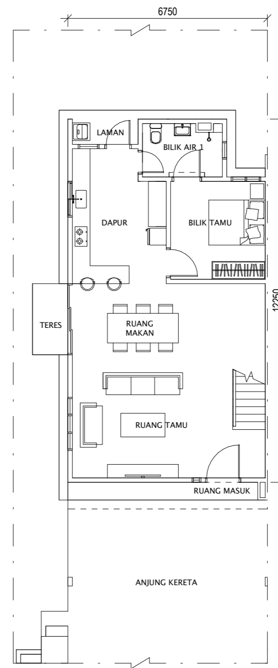
TINGKAT BAWAH
