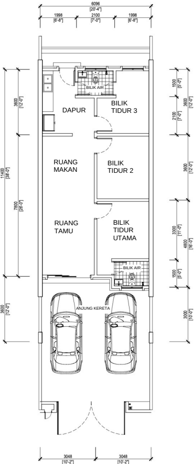
PELAN LANTAI TERES SETINGKAT
