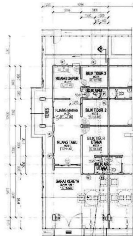
PELAN LANTAI
