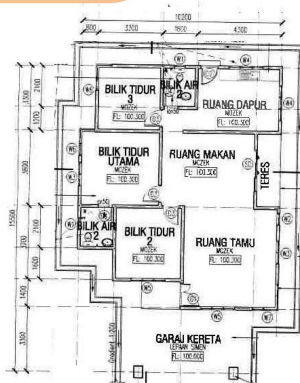
PELAN LANTAI
