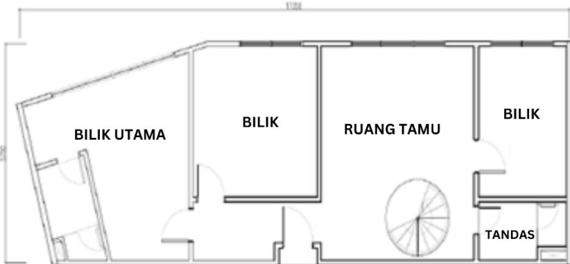
G2- Tingkat Bawah
