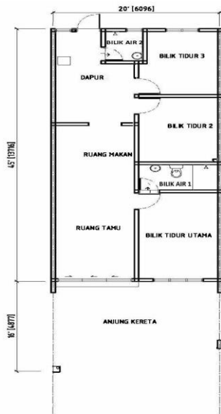
PELAN LANTAI
