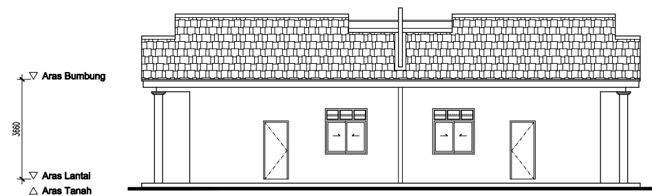
PANDANGAN BELAKANG
