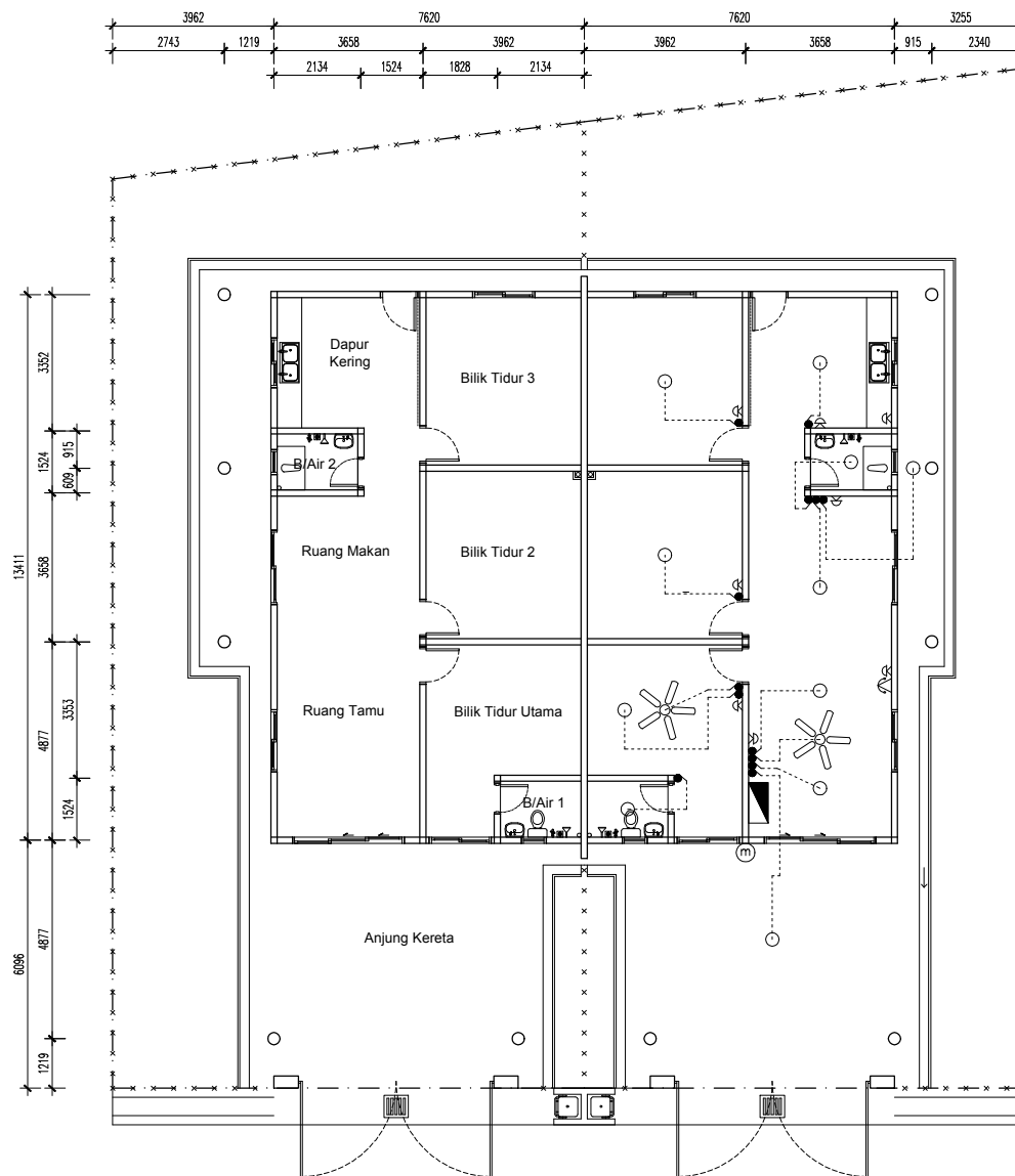
PELAN LANTAI
