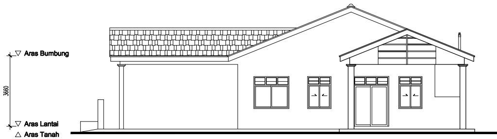
PANDANGAN KANAN
