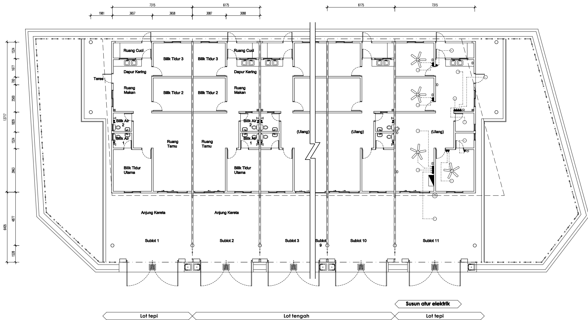
PELAN LANTAI
