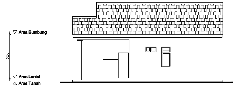
PANDANGAN BELAKANG
