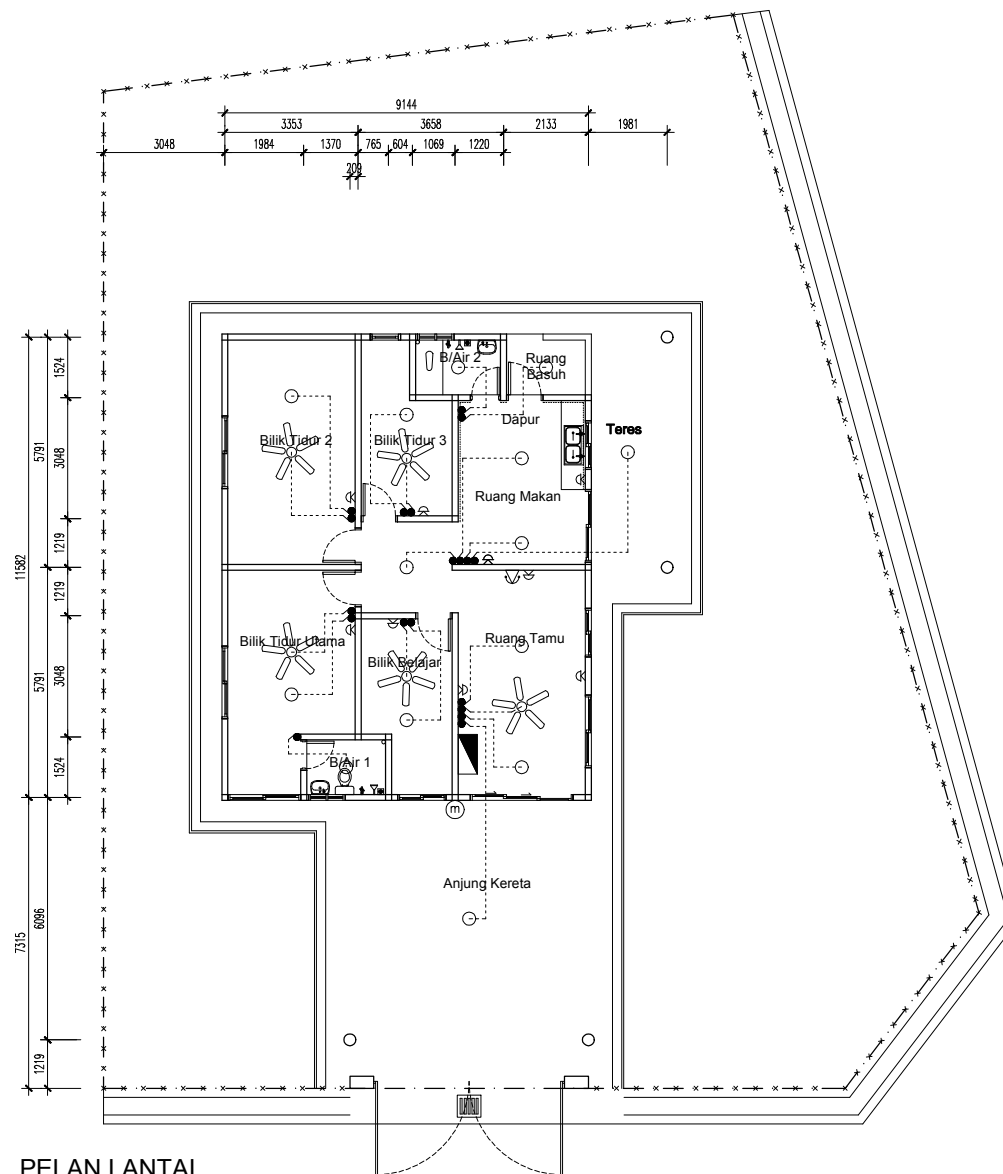
PELAN LANTAI
