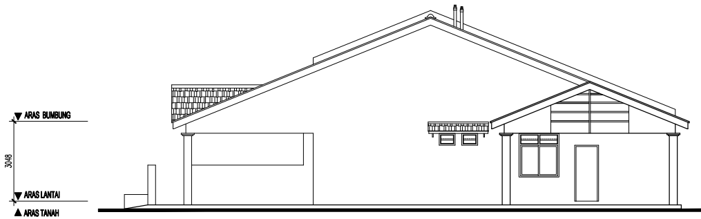
PANDANGAN KANAN
