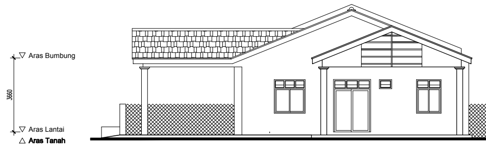
PANDANGAN SISI
