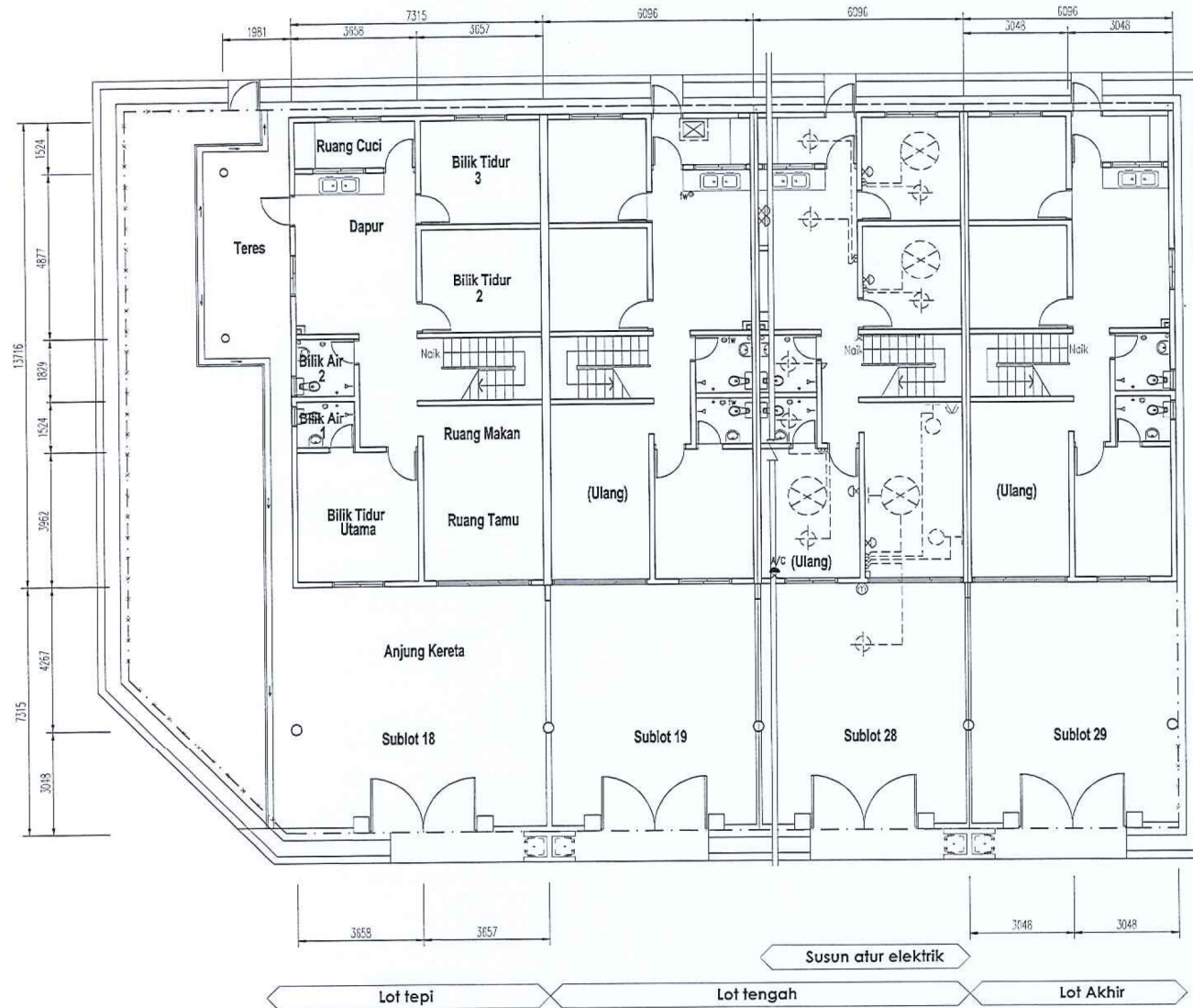
PELAN LANTAI
