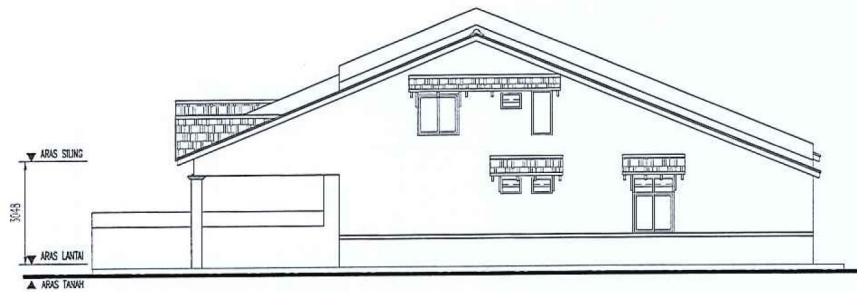
PANDANGAN KANAN
