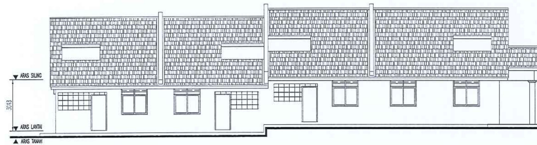
PANDANGAN BELAKANG
