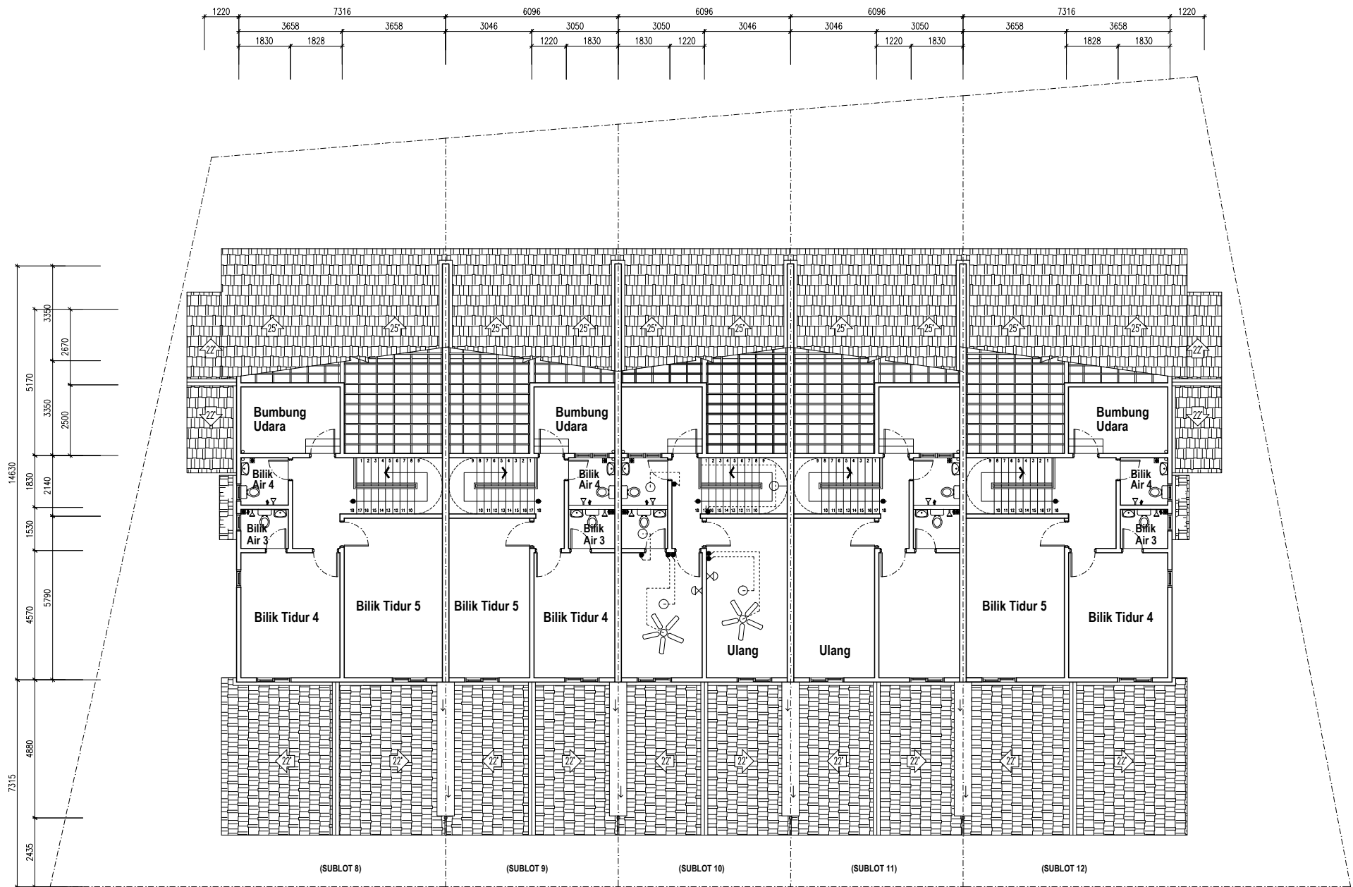
PELAN LANTAI ARAS 1
