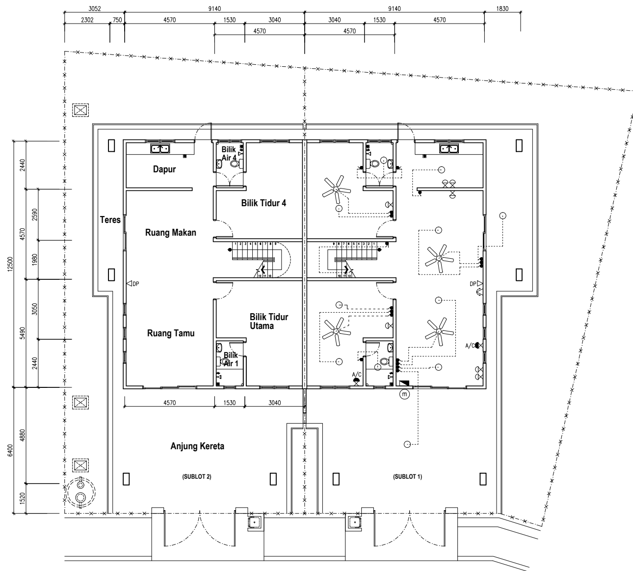
PELAN LANTAI ARAS TANAH
