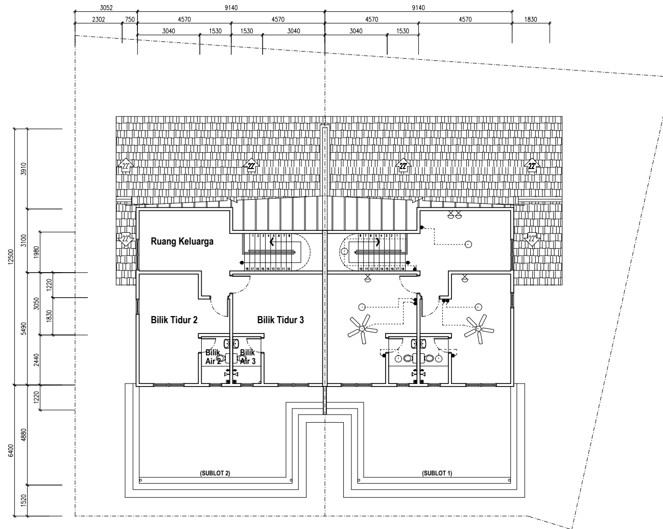
PELAN LANTAI ARAS 1
