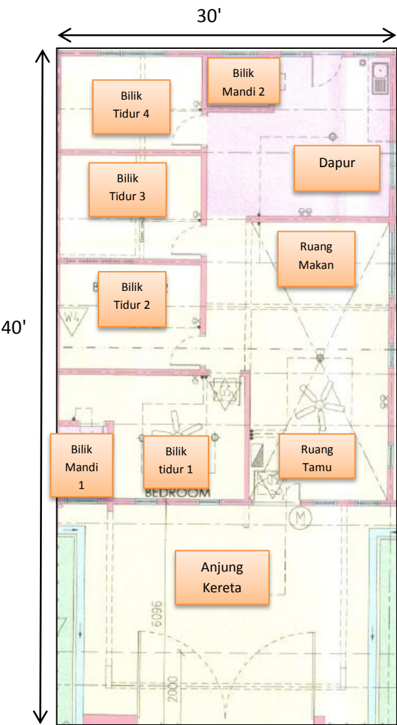
RUMAH BERKEMBAR SETINGKAT JENIS A
