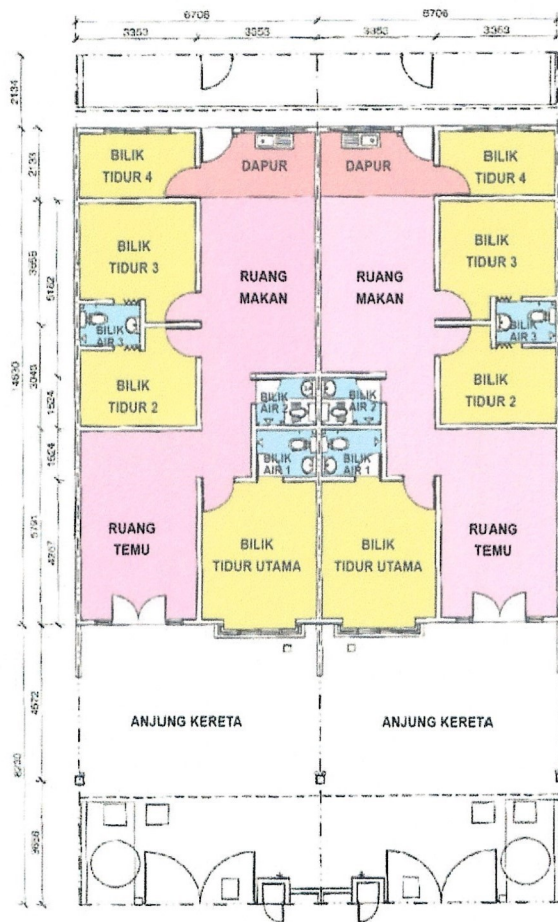
PELAN LANTAI
