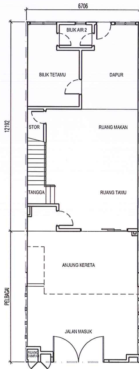
PELAN TINGKAT BAWAH
