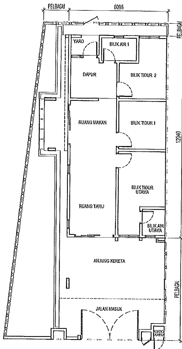
PELAN TINGKAT BAWAH
