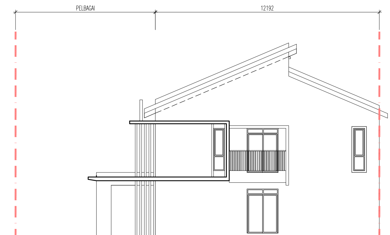
PANDANGAN SISI
