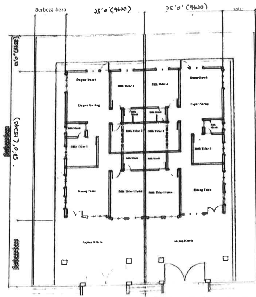
PELAN LANTAI
