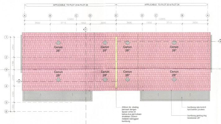
27. RUMAH BERKEMBAR - PELAN BUMBUNG SKALA: 1:100
