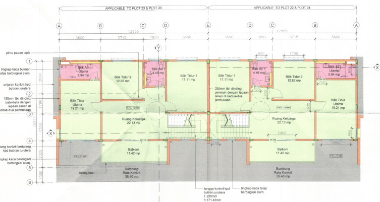
26. RUMAH BERKEMBAR - PELAN TINGKAT SATU SKALA: 1:100
