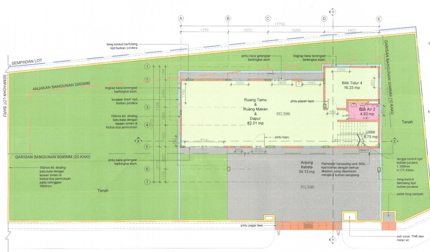
16 RUMAH BANGLO - PELAN TINGKAT BAWAH SKALA: 1:100
