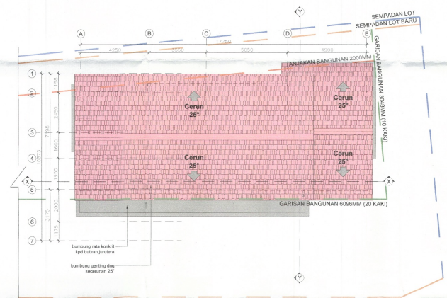
18 RUMAH BANGLO - PELAN BUMBUNG SKALA: 1:100
