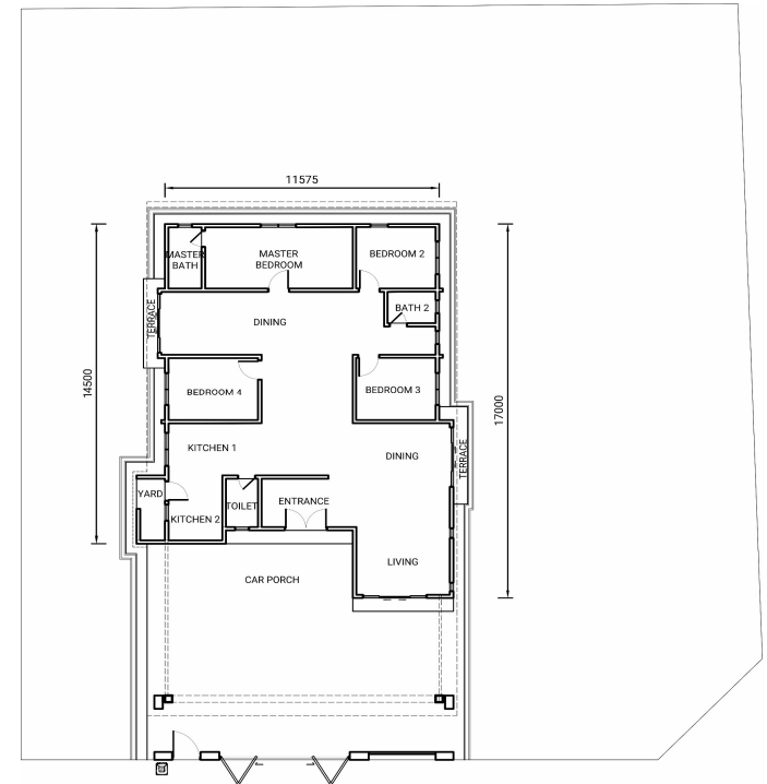
PELAN LANTAI
