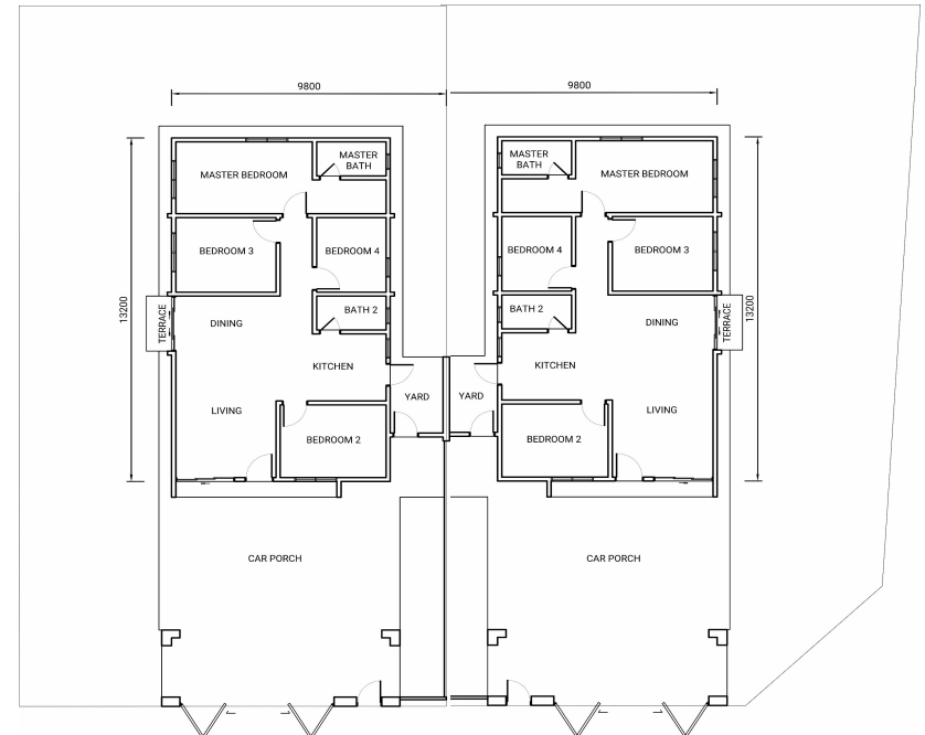
PELAN LANTAI
