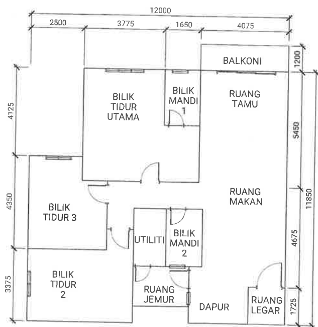
PELAN LANTAI
