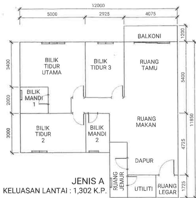
PELAN LANTAI
