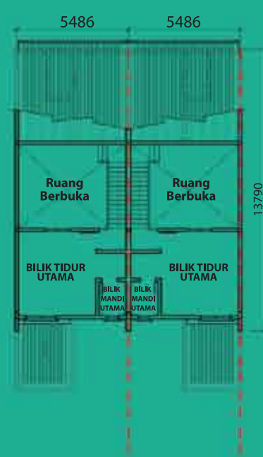
PELAN LANTAI ATAS
