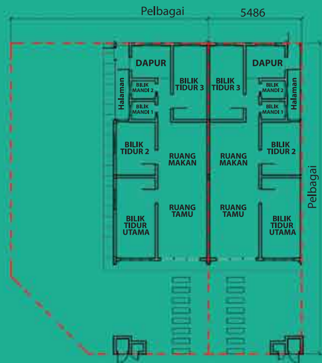
PELAN LANTAI BAWAH
