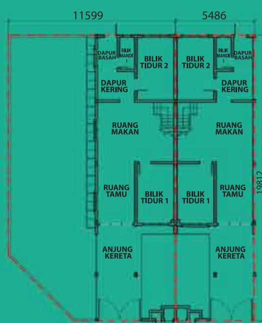
PELAN LANTAI BAWAH
