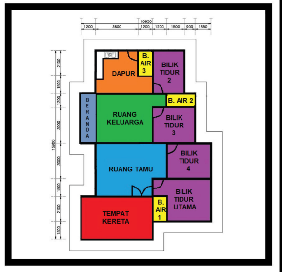
RUMAH BANGLO TYPE F
