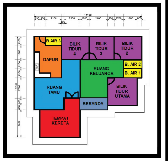
RUMAH BANGLO TYPE G
