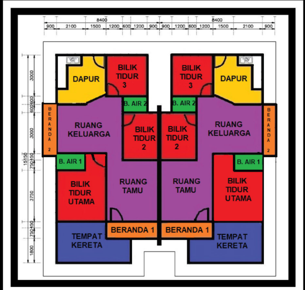
RUMAH BERKEMBAR TYPE B
