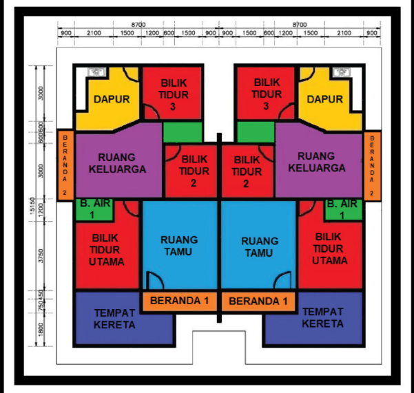
RUMAH BERKEMBAR TYPE A
