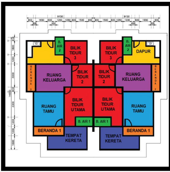
RUMAH BERKEMBAR TYPE C
