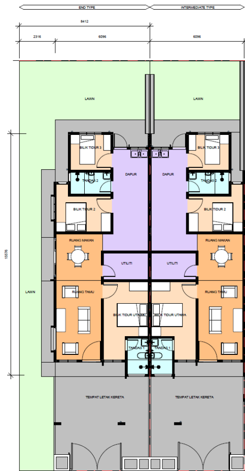
PELAN LANTAI
