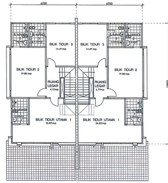
Pelan Lantai Atas
