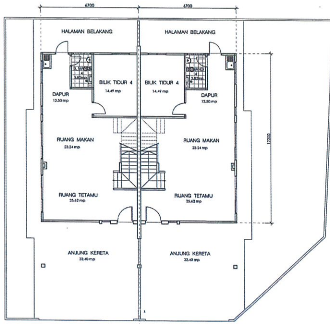
Pelan Lantai Bawah
